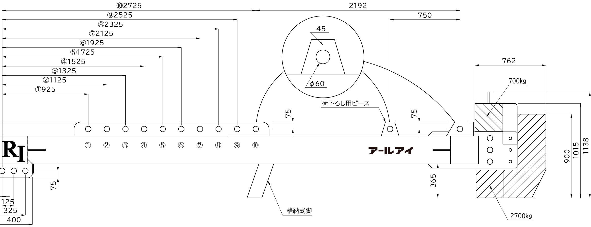
側面図
