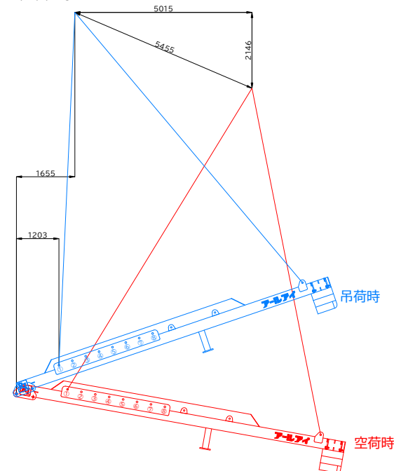
BBバランサー26000N 19.5t吊り概算変動図 BBバランサー26000N (標準仕様) 参考ワイヤ IWRCφ40×10m片アイ片シンプル 4本 ワイヤIWRCφ40 =吊り角度60°2点吊安全荷重30,000kg 概算総自重 27.073ton (BB26000概算総自重7,573kg+吊り荷19,500kg) 参考シャックル 強力長シャックル 20t×4個 吊り位置 ①
