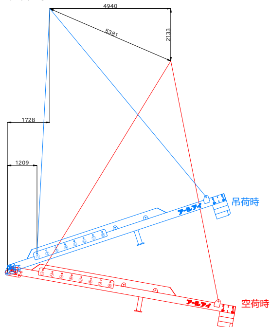
BBバランサー26000N 18.5t吊り概算変動図 BBバランサー26000N (標準仕様) 参考ワイヤ IWRCφ38×10m片アイ片シンプル 4本 ワイヤIWRCφ38 =吊り角度60°2点吊安全荷重27,100kg 概算総自重 26.073ton (BB26000概算総自重7,573kg+吊り荷18,500kg) 参考シャックル 強力長シャックル 20t×4個 吊り位置 ①
