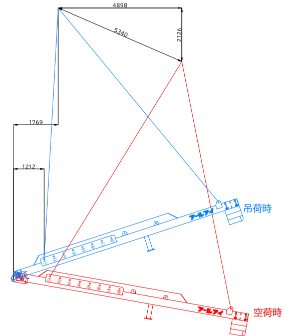
BBバランサー26000N 18t吊り概算変動図 BBバランサー26000N (標準仕様) 参考ワイヤ IWRCφ38×10m片アイ片シンプル 4本 ワイヤIWRCφ38 =吊り角度60°2点吊安全荷重27,100kg 概算総自重 25.573ton (BB26000概算総自重7,573kg+吊り荷18,000kg) 参考シャックル 強力長シャックル 20t×4個 吊り位置 ①
