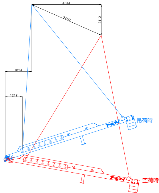
BBバランサー26000N 17t吊り概算変動図 BBバランサー26000N (標準仕様) 参考ワイヤ IWRCφ38×10m片アイ片シンプル 4本 ワイヤIWRCφ38 =吊り角度60°2点吊安全荷重27,100kg 概算総自重 24.573ton (BB26000概算総自重7,573kg+吊り荷17,000kg) 参考シャックル 強力長シャックル 20t×4個 吊り位置 ①
