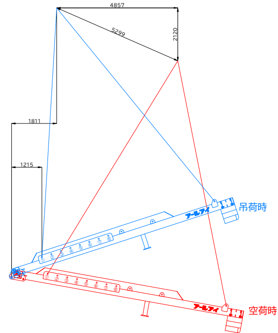
BBバランサー26000N 17.5t吊り概算変動図 BBバランサー26000N (標準仕様) 参考ワイヤ IWRCφ38×10m片アイ片シンプル 4本 ワイヤIWRCφ38 =吊り角度60°2点吊安全荷重27,100kg 概算総自重 25.073ton (BB26000概算総自重7,573kg+吊り荷17,500kg) 参考シャックル 強力長シャックル 20t×4個 吊り位置 ①
