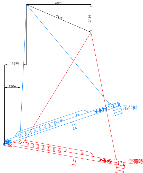
BBバランサー26000N 19t吊り概算変動図 BBバランサー26000N (標準仕様) 参考ワイヤ IWRCφ40×10m片アイ片シンプル 4本 ワイヤIWRCφ40 =吊り角度60°2点吊安全荷重30,000kg 概算総自重 26.573ton (BB26000概算総自重7,573kg+吊り荷19,000kg) 参考シャックル 強力長シャックル 20t×4個 吊り位置 ①
