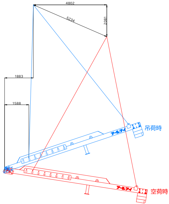
BBバランサー26000N 16.5t吊り概算変動図 BBバランサー26000N (標準仕様) 参考ワイヤ IWRCφ38×10m片アイ片シンプル 4本 ワイヤIWRCφ38 =吊り角度60°2点吊安全荷重27,100kg 概算総自重 24.073ton (BB26000概算総自重7,573kg+吊り荷16,500kg) 参考シャックル 強力長シャックル 14t×4個 吊り位置 ②
