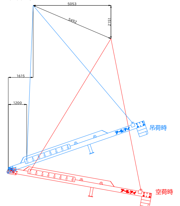
BBバランサー26000N 20t吊り概算変動図 BBバランサー26000N (標準仕様) 参考ワイヤ IWRCφ40×10m片アイ片シンプル 4本 ワイヤIWRCφ40 =吊り角度60°2点吊安全荷重30,000kg 概算総自重 27.573ton (BB26000概算総自重7,573kg+吊り荷20,000kg) 参考シャックル 強力長シャックル 20t×4個 吊り位置 ①
