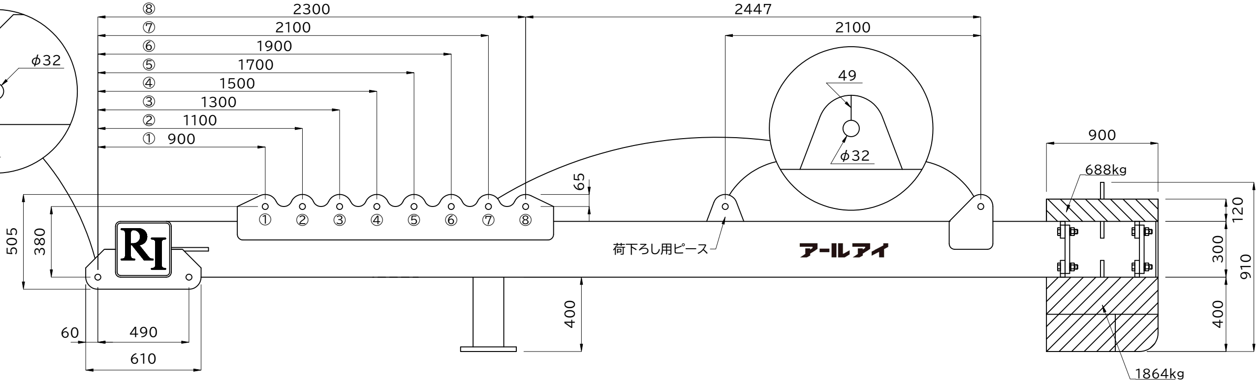
側面図
